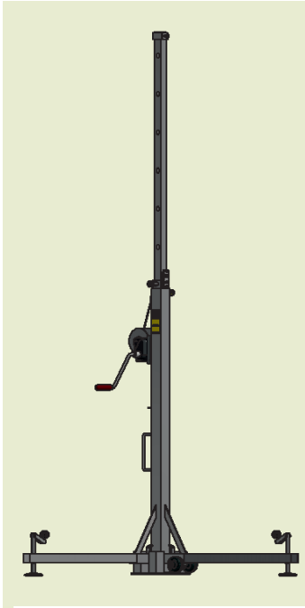
Schieben Sie den ersten Abschnitt der Turm hoch.
